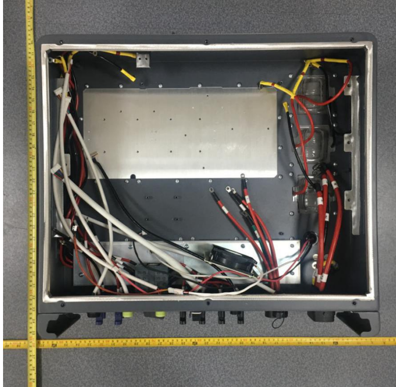
Fig. 13 (HYD 10-20KTL-3PH Empty case)
